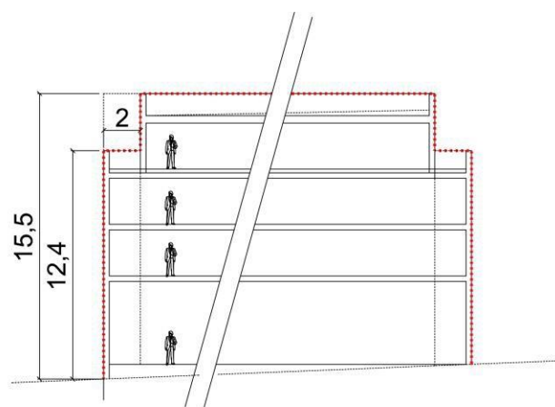
TOITURE TERRASSE
